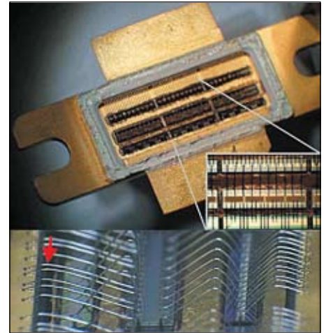
Рис. 2. Вид LDMOS-транзистора со снятой крышкой (фрагмент соединительных проводников, используемых в транзисторе, увеличен; красной стрелкой отмечены проводники наиболее подверженные обрыву из-за усталости материала)
